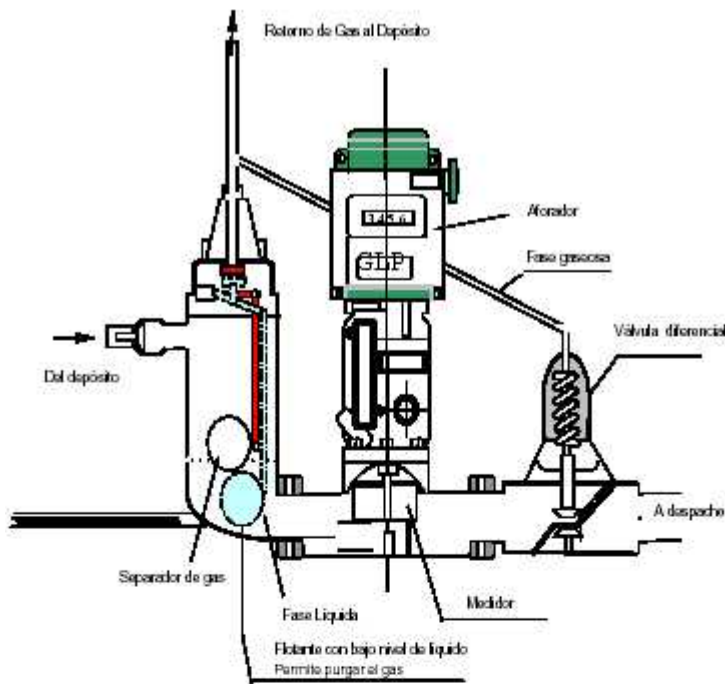
Figura 4: ESQUEMA TIPO DE SEPARADOR DE FASE GASEOSA
