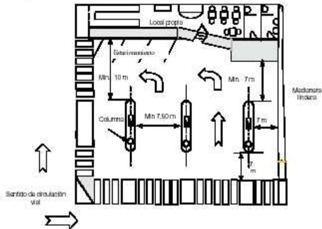
Figura N° 6 Tipo de ubicación en estación de carga cautiva
